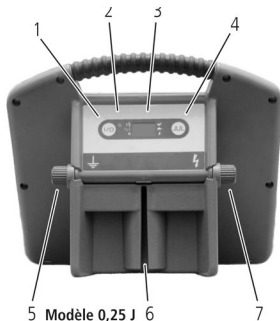
Modèle 0,25 J 6
